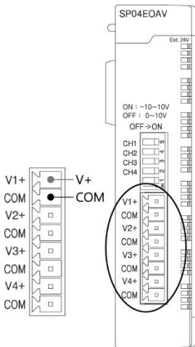
▶ SP04EOAV 전압 출력
