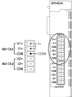
▶ SP04EAA(-A, -E) 전류 입력
