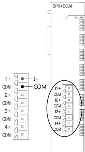
▶ SP04EOAI 전류 출력
