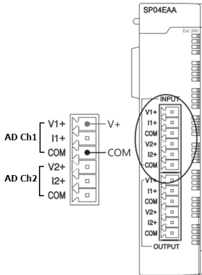
▶ SP04EAA(-A, -E) 전압 입력
