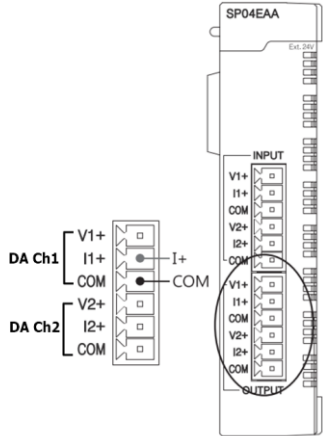
▶ SP04EAA(-A, -E) 전류
