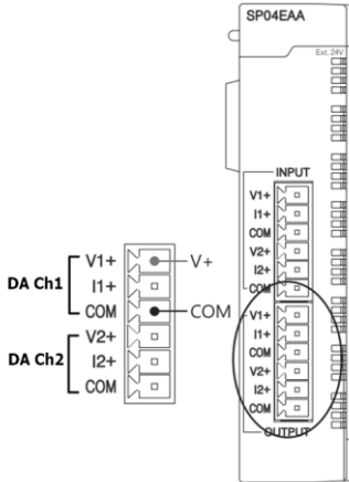
▶ SP04EAA(-A, -E) 전압 출력
